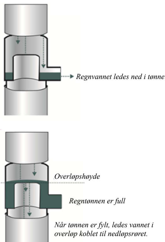
Regntønne med overløp. Illustrasjon: SLA
