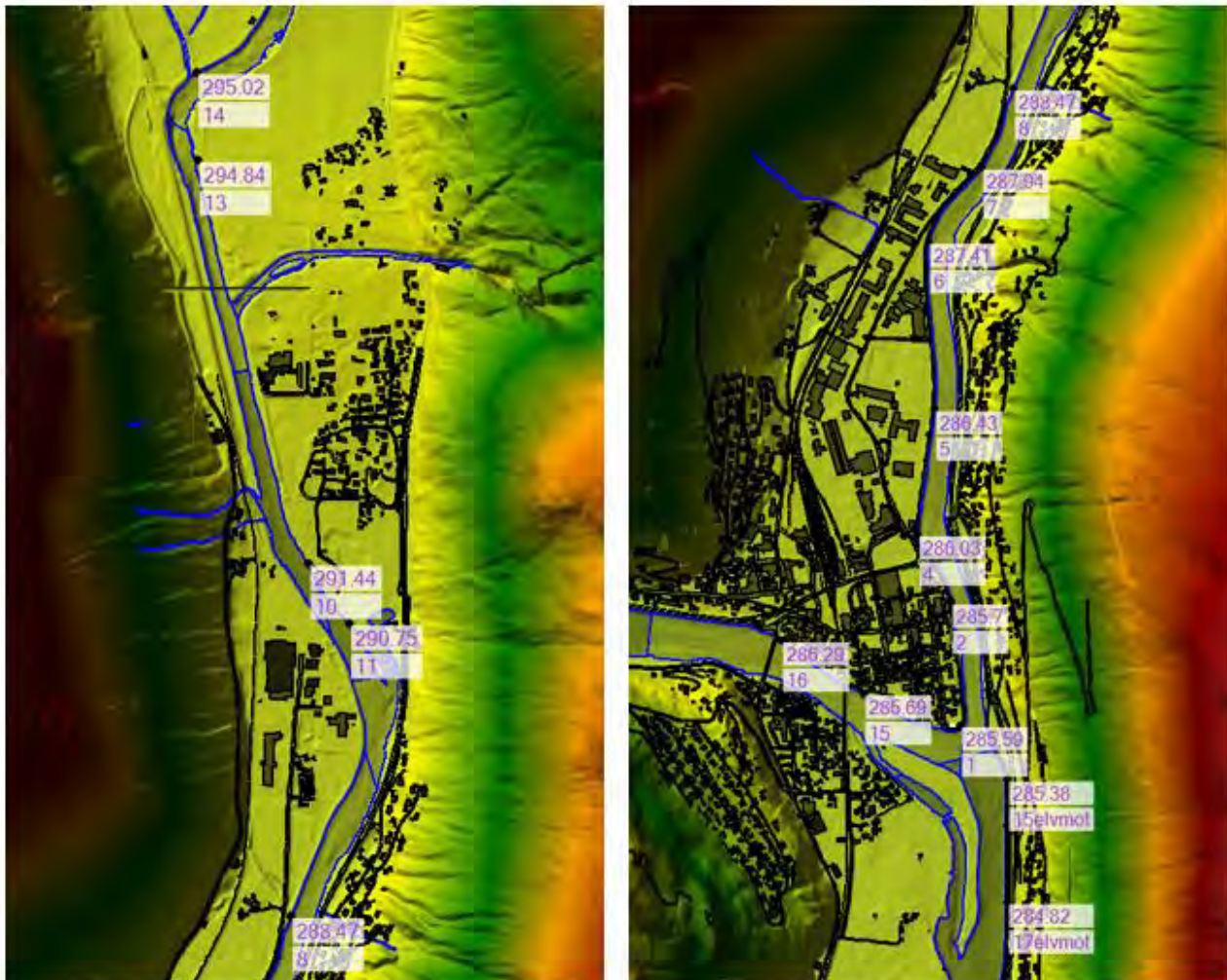
Figur 5 Oversiktskart med punkt hvor vannstand er innmålt av Rondane Oppmåling under ekstremværet «Hans», 10. august 2023 (dagen etter kulminasjonsvannføring i Rosten). Innmålt vannnivå og punktnr. er oppgitt med lilla tekst for hvert innmålingspunkt. Punkt 10 og 14 i venstre bilde ligger oppstrøms Ula.
