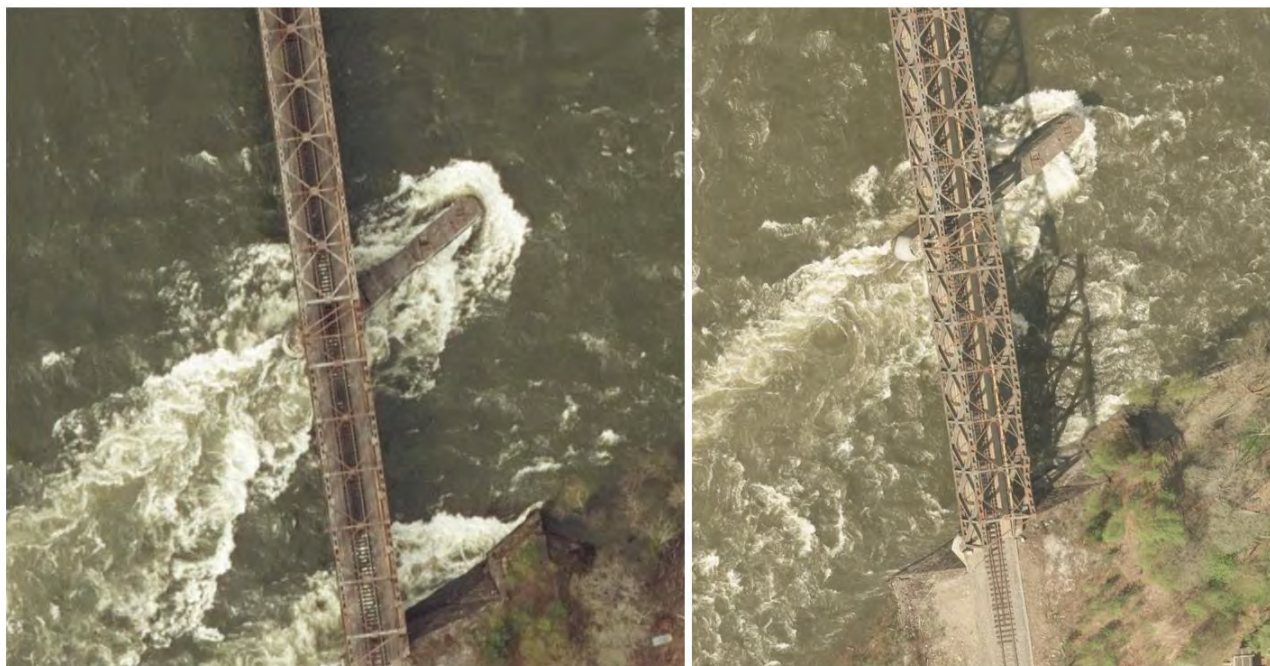
Figur 23 Flyfoto av Sjoa jernbanebru ved flom i 2018 (venstre) og 2013 (høyre). Foto fra www.norgebilder.no .
