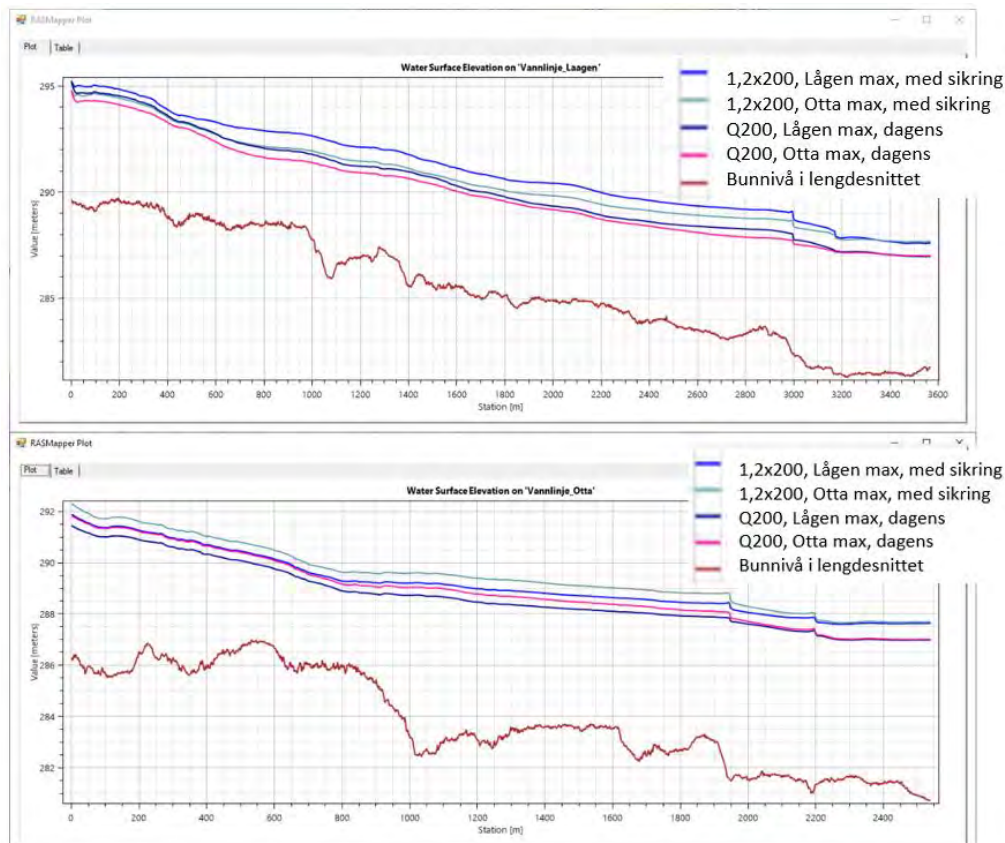
Figur 39 Vannlinje i Lågen (øverst) og Otta (nederst) – sammenlikning av vannstand ved Q 200 i dagens situasjon mot 1,2xQ 200 med flomsikring. Vannlinjenes plassering er vist i Figur 37 og Figur 38.
