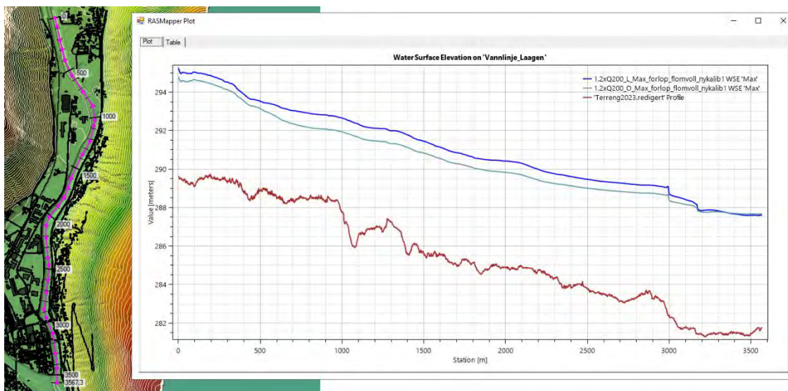
Figur 37 Vannlinje i Lågen ved 1,2xQ 200 med sikring for belastningstilfelle 1 (kulminasjonsflom i Lågen, blå linje) og 2 (kulminasjonsflom i Otta, grønn linje). Rød kurve viser elvebunnens nivå.
