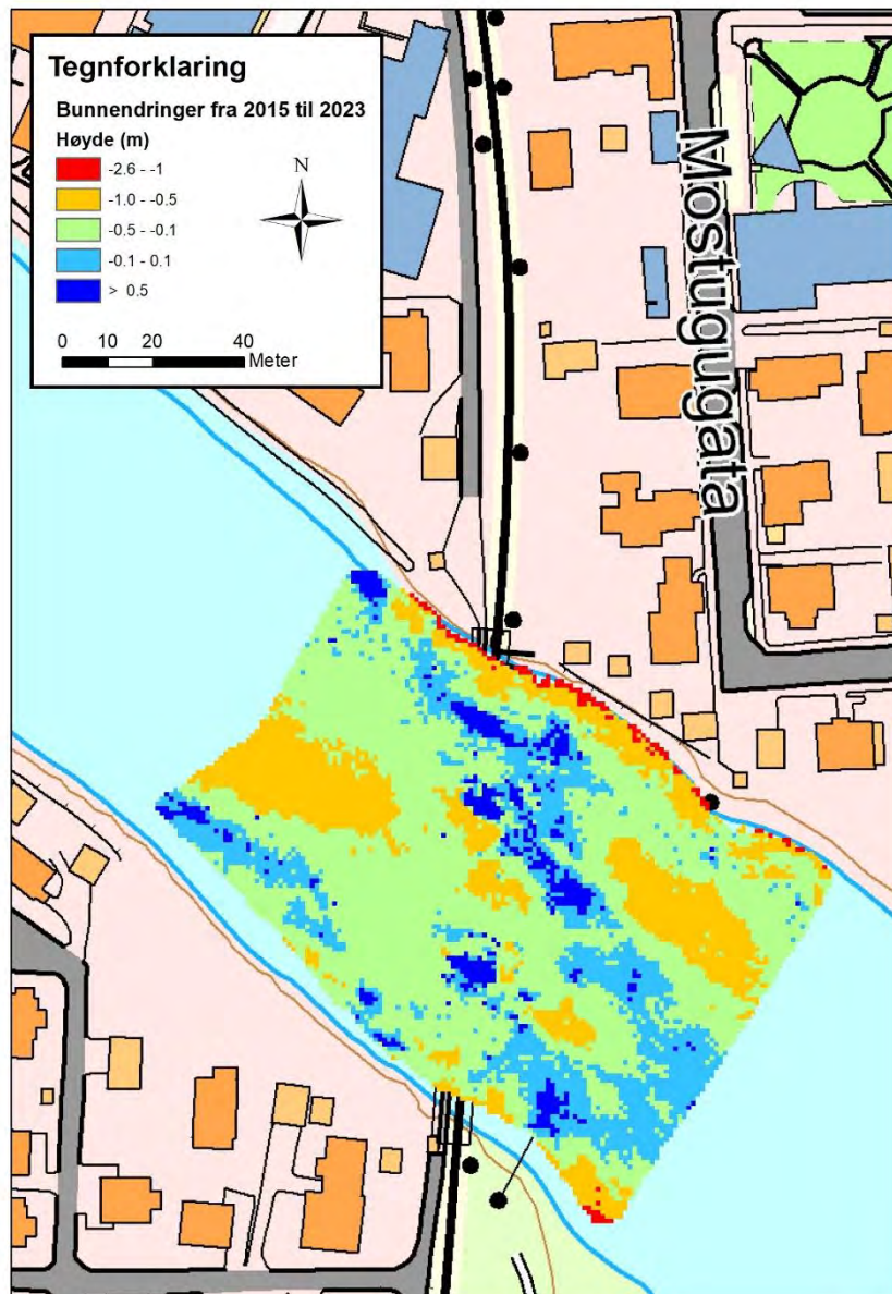
Figur 16 Endringer i elvebunnen ved Otta jernbanebru mellom 2015 og 2023. Høydeforskjellene er beregnet mellom ekkolodding-2023 (mottatt fra BaneNOR) sammenlignet med bunnkartlegging fra 2015 (hentet fra høydedata). Negative verdier tilsvarer bunnsenkning (rød, oransje og lysgrønn farge)
