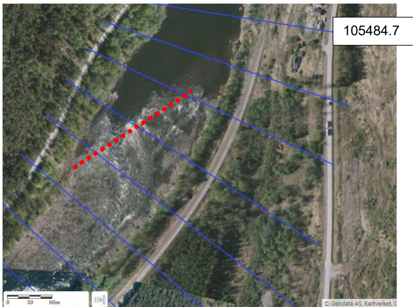
Figur 30 Stryk mellom Sjoa jernbanebru og Sjoa tettsted. Det mangler dybde data i området. Blå linjer er tverrsnitt fra 2017-modellen, med stipulert/regelbasert geometri. Ved 1,2xQ_{200} gir oppdatert 1D-modell at strømmingen går gjennom kritisk i tverrsnitt 105484.7. Rød, stiplet linje antyder naturlig terskel av stein som kan sees fra flyfoto. Foto fra www.norgebilder.no .
