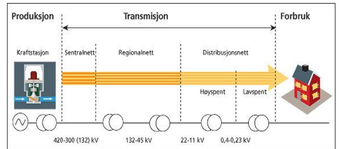
Figur 2 Skjematisk oppbygging av kraftsystemet (kjelde NVE)
